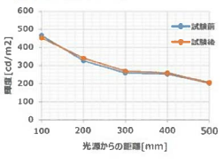
耐寒性 : R.T.→40℃×500h→R.T.
