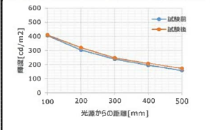
ヒートサイクル : R.T.→80℃・90%×2h→R.T.→30℃×2h→R.T. (1019/9%)
