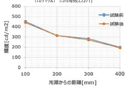
塩水噴霧 : 塩水噴霧: 35℃・47%×8h→凍結: 35℃・47%×16h (109/9%) ※JIS電機(22374)
